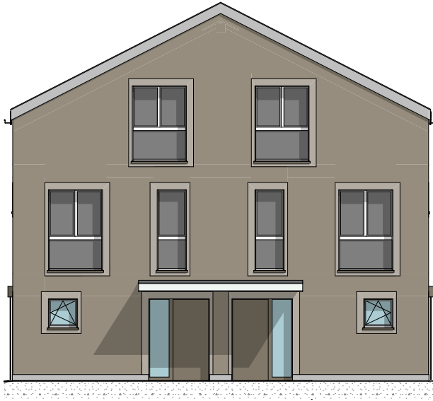
Nordfassade
